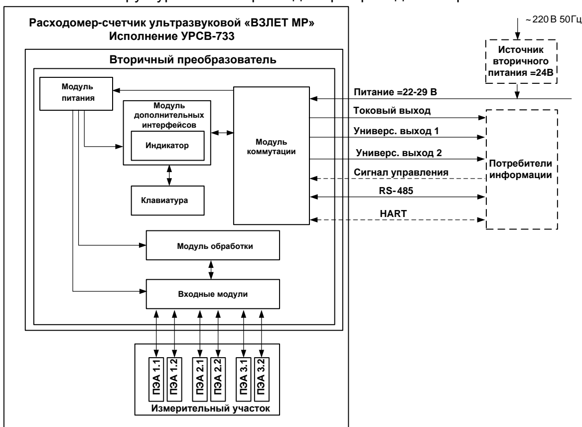
Рис.2. Структурная схема расходомера.
