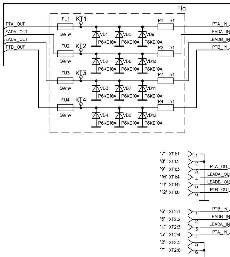
Рис. В.2. Блок БИЗ-11
