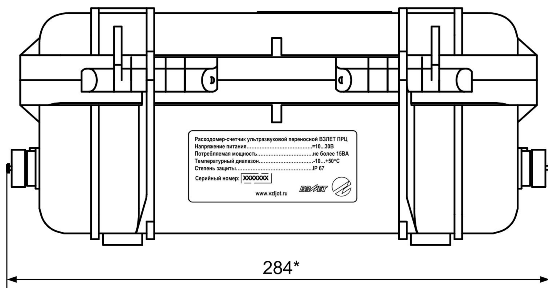
а) вид со стороны крышки
