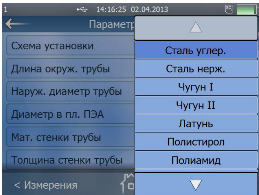
Рис.7. Пример индикации выбора списочных параметров в подменю «Мат. стенки трубы» меню «Параметры трубы»
