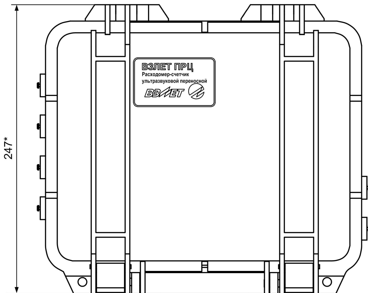
а) вид со стороны крышки
