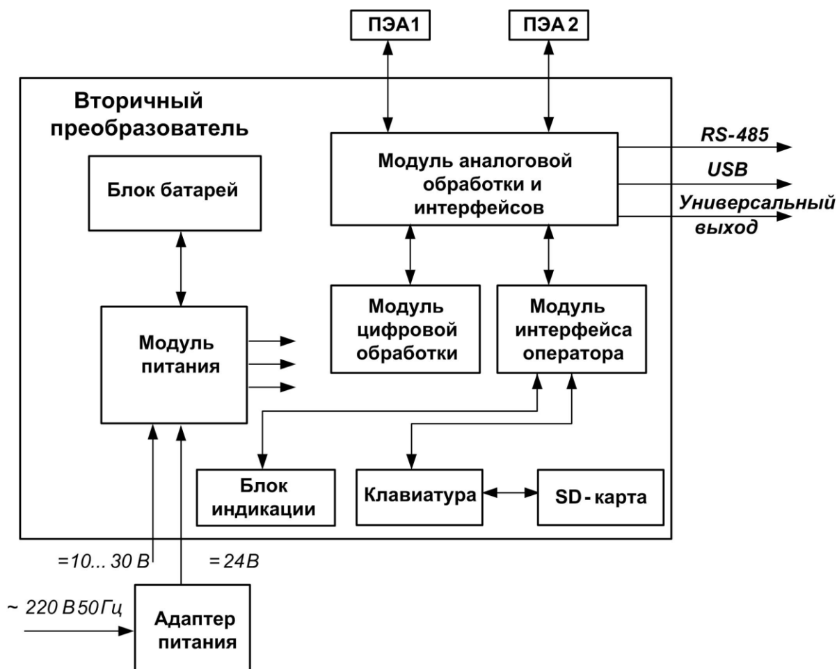
Рис.3. Структурная схема расходомера.
