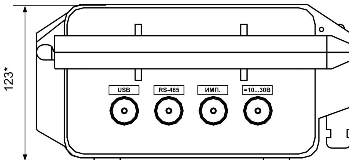
в) вид со стороны разъемов питания и связи
