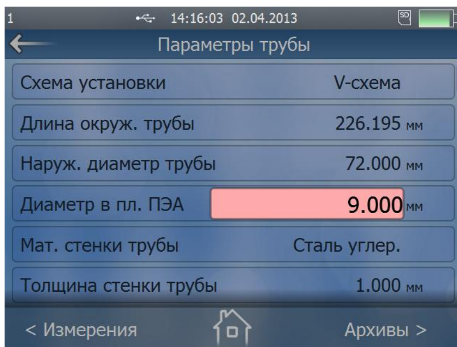
Рис.6. Ошибочно введенное цифровое значение параметра «Диаметр в пл. ПЭА»
