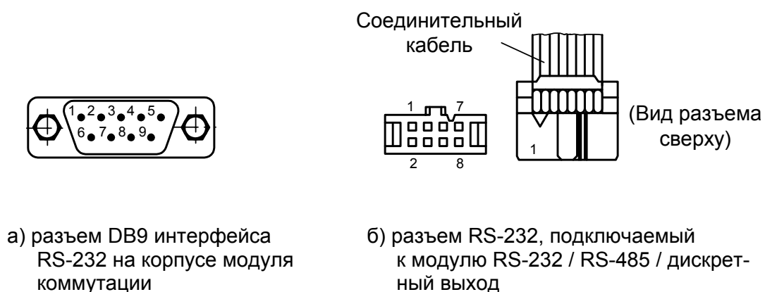
Рис.А.4. Разъемы кабеля интерфейса RS-232.
