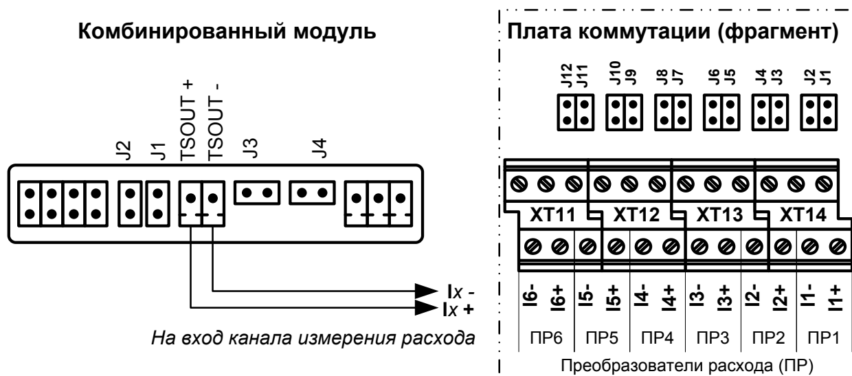
Рис.К.3. Схема подключения при проверке канала измерения расхода.
