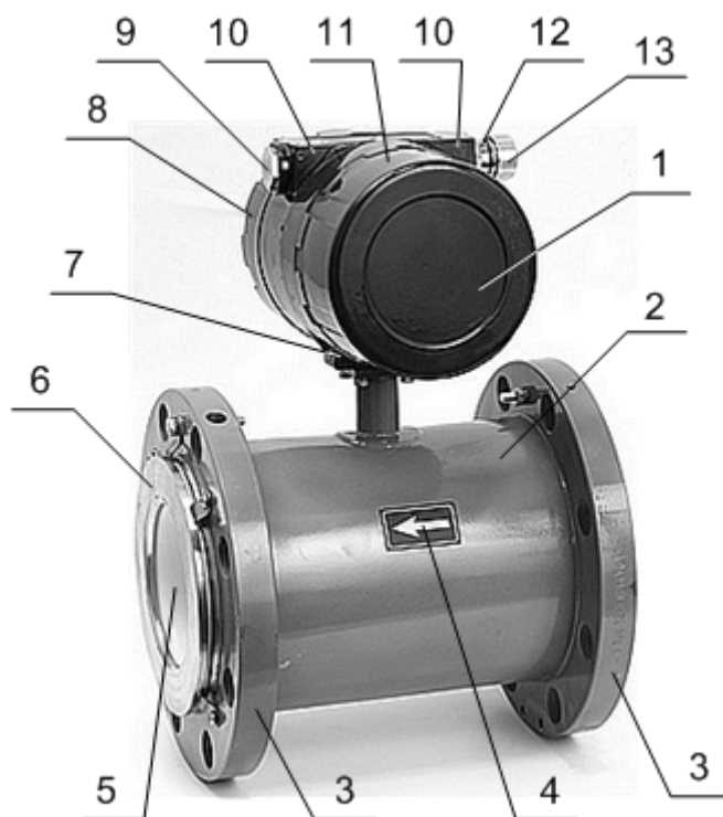
Рис.1. Внешний вид расходомера ВЗЛЕТ ТЭР.
