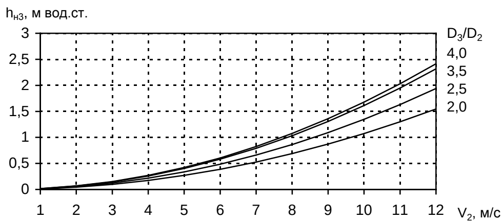
Рис.4. Графики зависимостей потерь напора в конфузоре (а), прямолинейном участке (б) и диффузоре (в).
