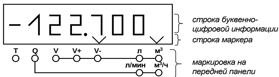
Рис.2. Вид индикатора расходомера и маркировки обозначений на передней панели при индикации объема обратного потока (значение V- = -122,7 м³).
