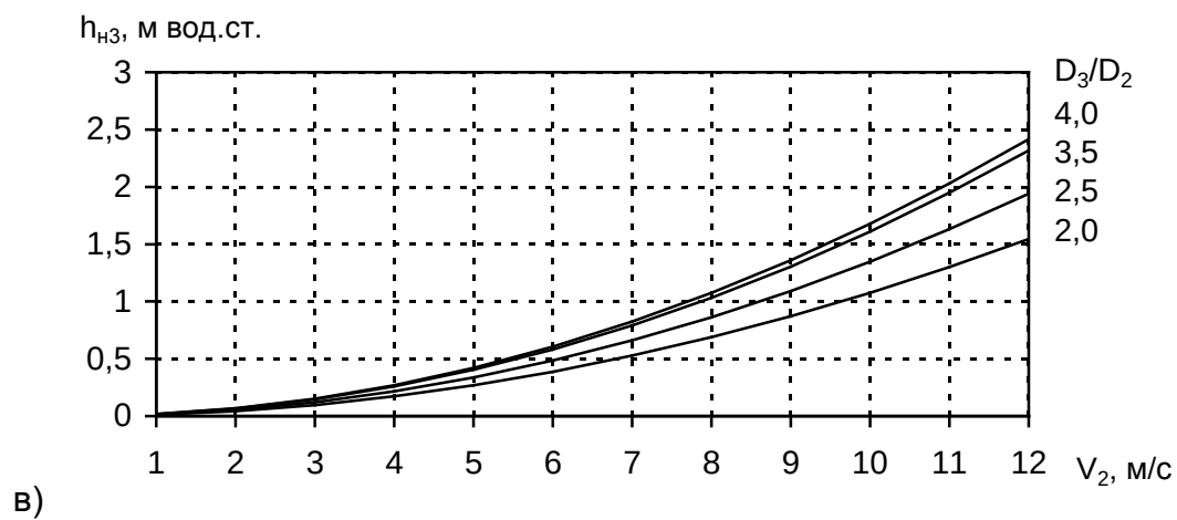
Рис. В.2. Графики зависимостей потерь напора в конфузоре (а), прямом участке (б) и диффузоре (в).
