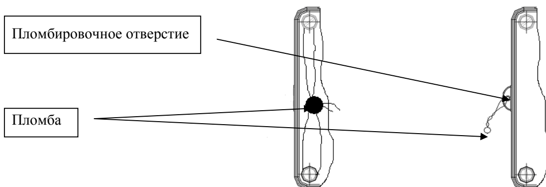
Рисунок. 2 - Схема пломбировки теплосчетчиков - регистраторов «ВЗЛЕТ ТСР-М»
