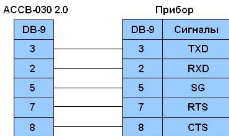
Рис.5. Подключение прибора по интерфейсу RS-232.
