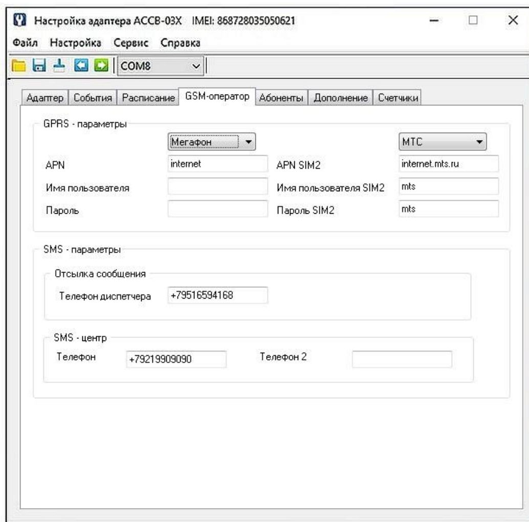
Рис.11. Вид вкладки «GSM-оператор».
