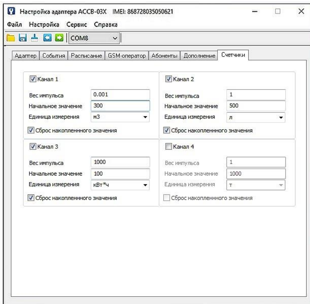
Рис.14. Вид вкладки «Счетчики».
