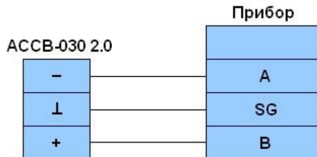
Рис.6. Подключение прибора по интерфейсу RS-485.
