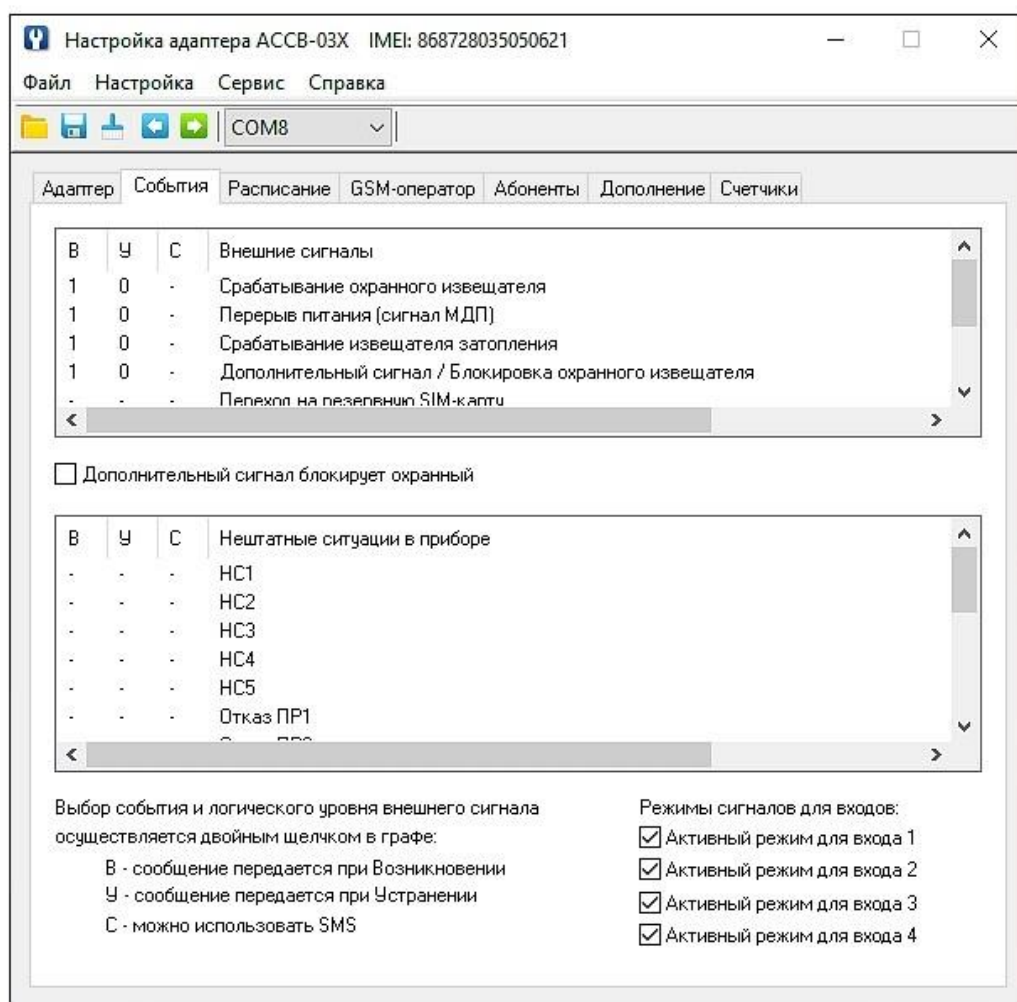
Рис.9. Вид вкладки «События».
