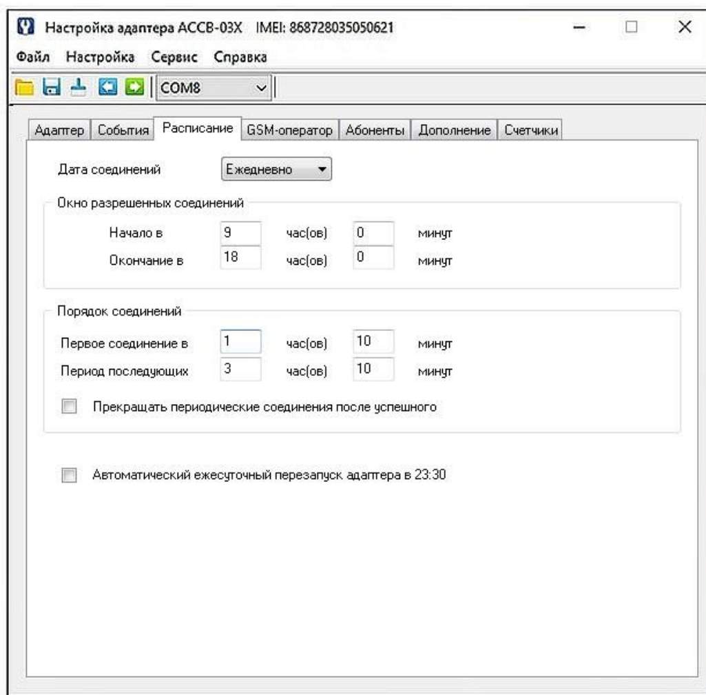
Рис.10. Вид вкладки «Расписание».
