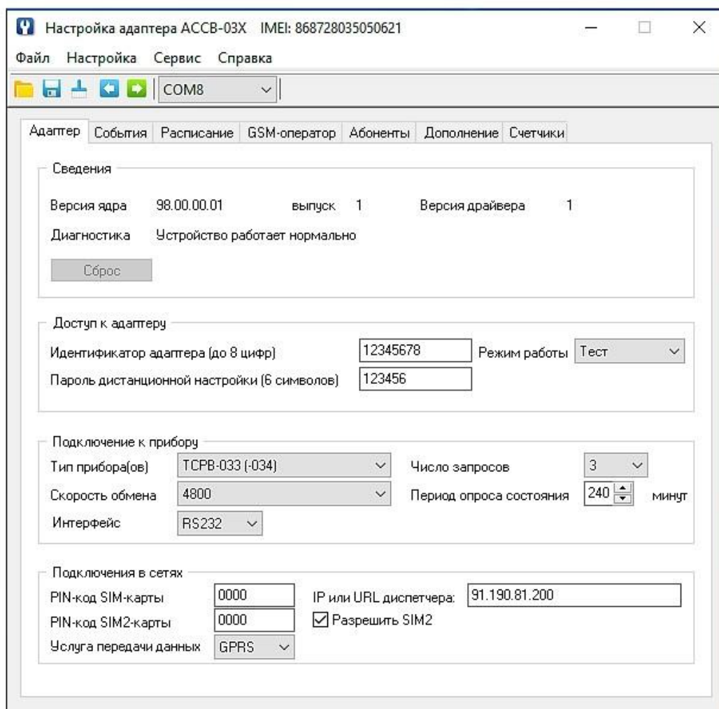
Рис.8. Вид основного окна программы настройки адаптера.
