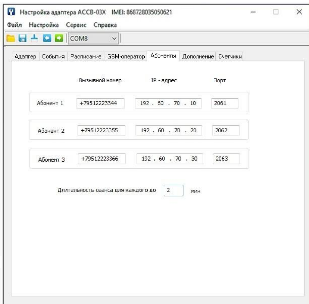
Рис.12. Вид вкладки «Абоненты».
